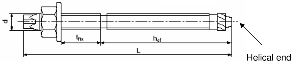
anchor rod
